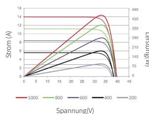
Strom-Spannungs- und Leistungs-Spannungs-Diagramme(445W)
