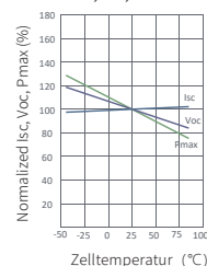
Temperaturabhängigkeit von I_{sc} , V_{oc} , P_{max}
